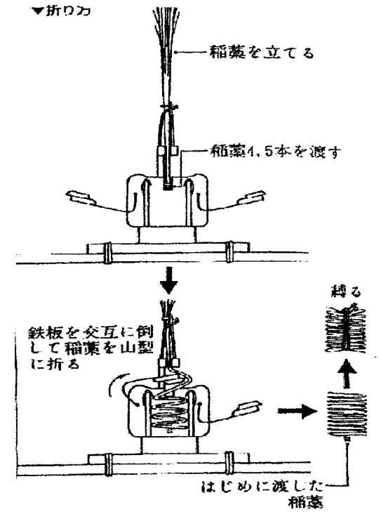
▲まぶし折機 まぶしを作る。明治末から使われる。
